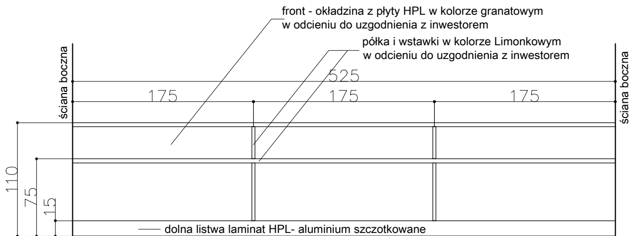
Widok zabudowy od strony komunikacji.
