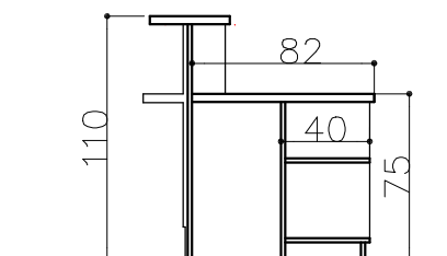
Przekrój - szafka z półką przestawną pod blatem.
