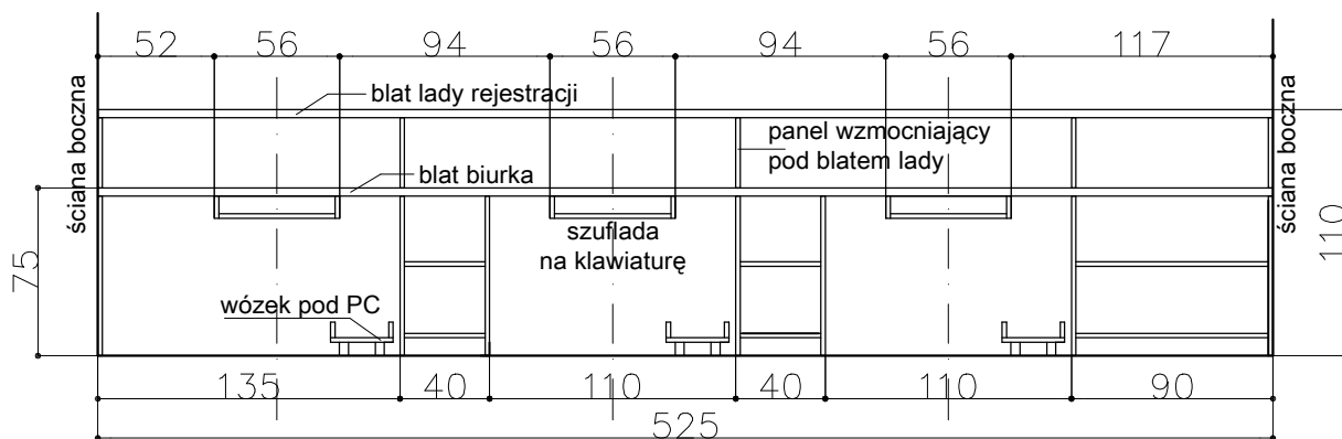
Widok od strony pracowników.
