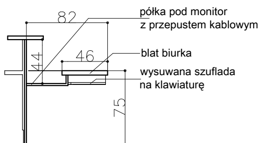
Przekrój - półka pod monitor z przepustem kablowym.
