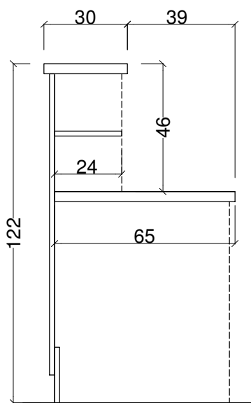
Przekrój przez biurko z ladą i półką.
